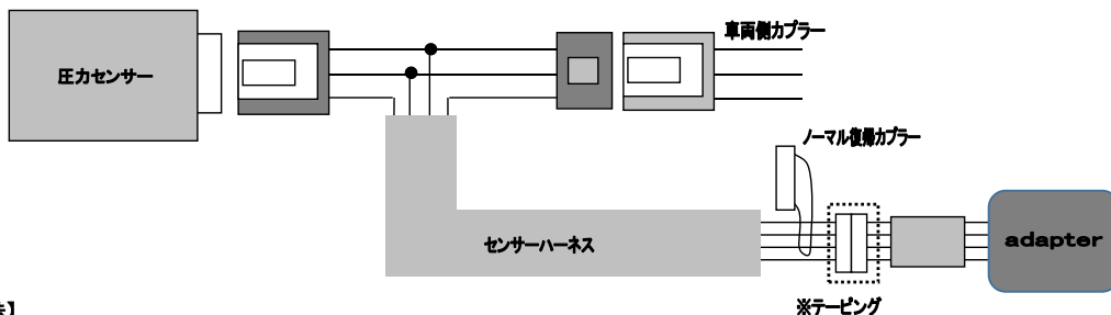
接続図
